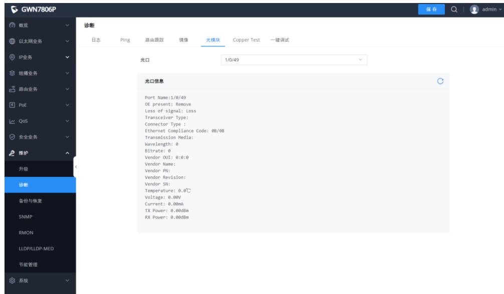
图 117 诊断-光模块
