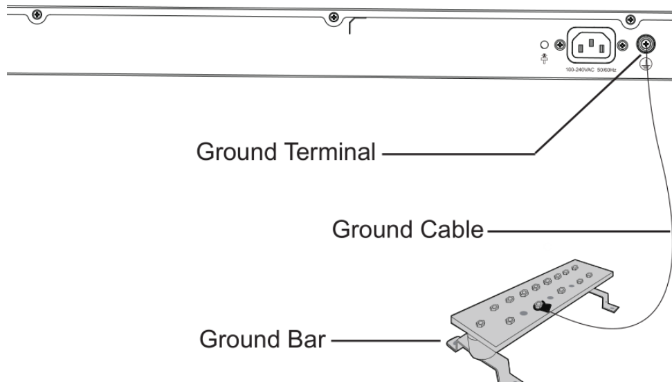
图 5 交换机接地
