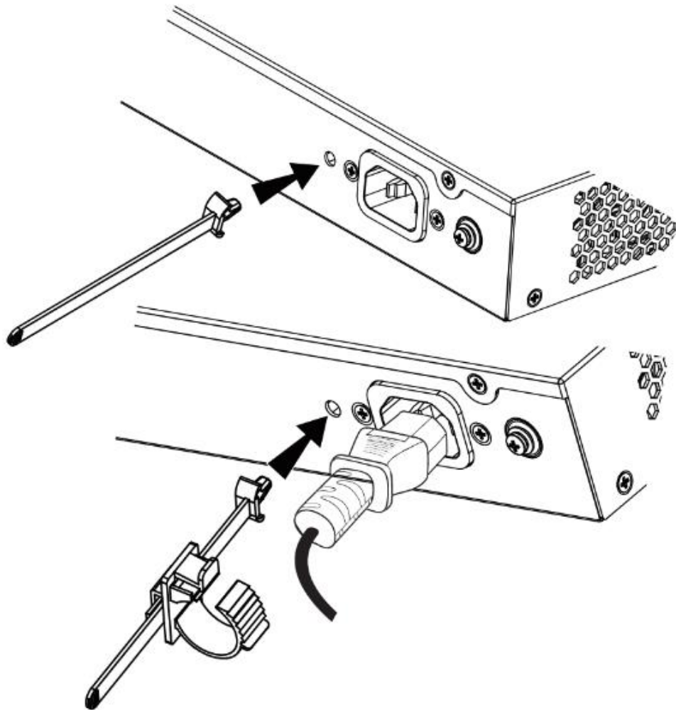
图 7 连接电源线防跳闸（可选）
