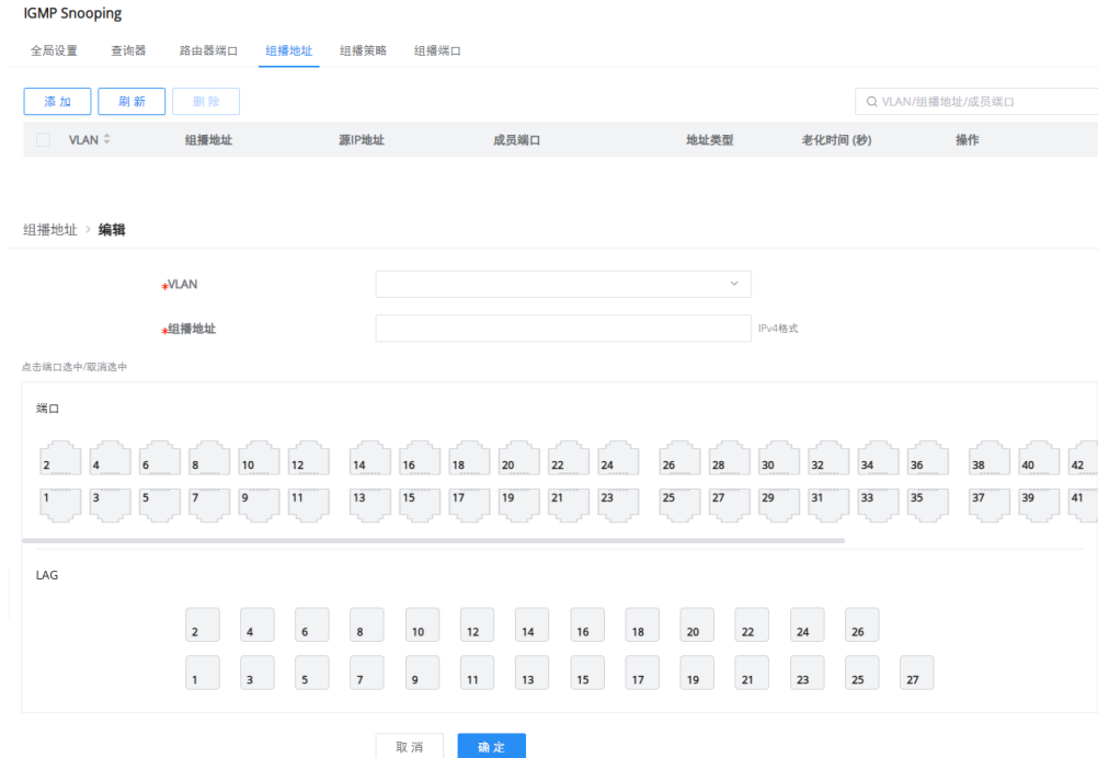
图 63 IGMP Snooping-组播地址
