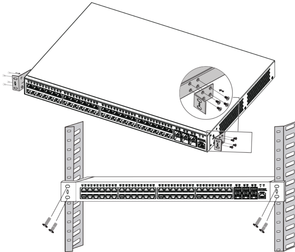
图 4 GWN7806(P) 机架安装
