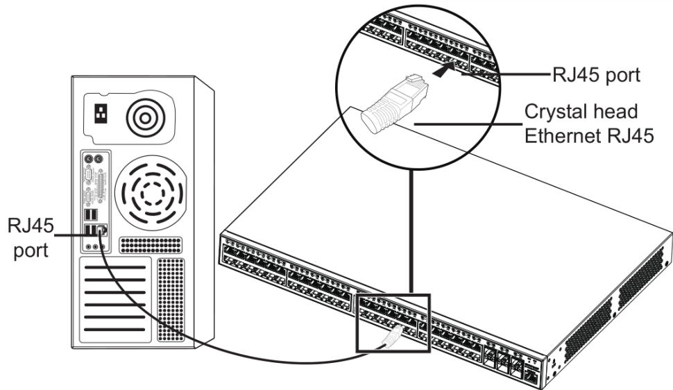
图 8 连接 RJ45 接口
