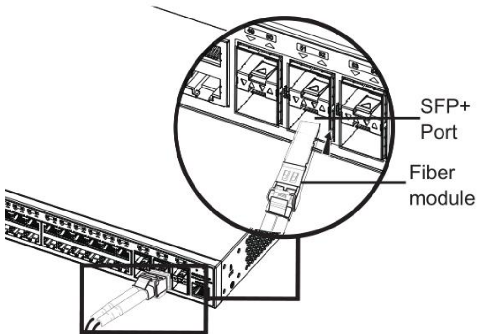
图 9 连接 SFP 接口
