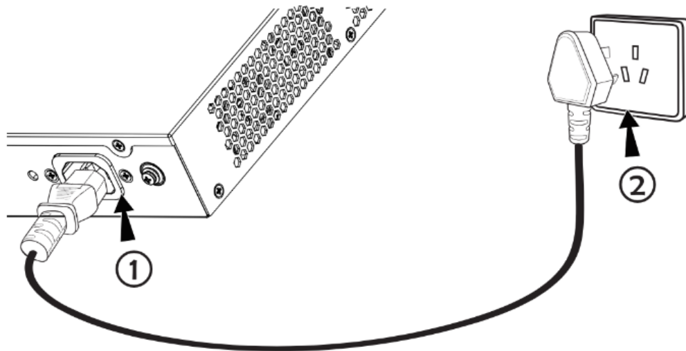
图 6 交换机上电
