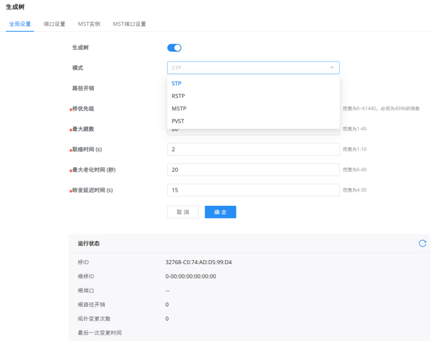
图 34 生成树-全局设置
