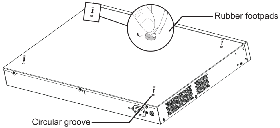
图 3 GWN7806(P)桌面安装
